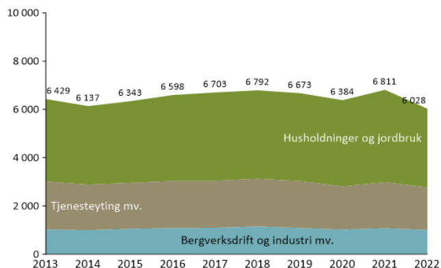
Figur 14: Utvikling i kraftforbruket i Innlandet
