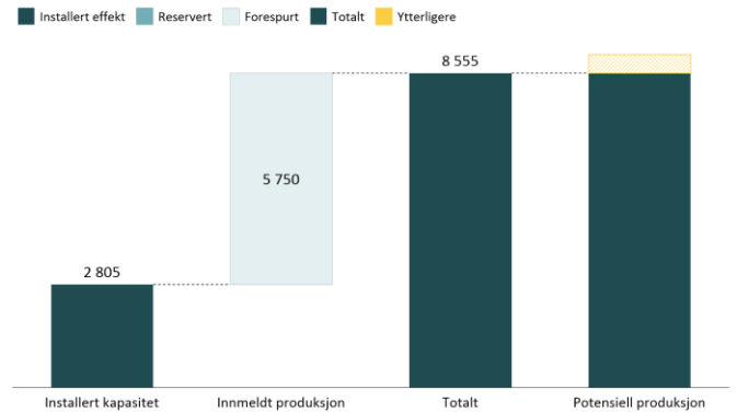
Figur 27: Tilknytningssaker hos Elvia (Innlandet) til produksjon (MW). Potensiell produksjon er inkludert ytterligere prosjekter som enda ikke er meldt til NVE eller Statnett, men som aktører ser på
